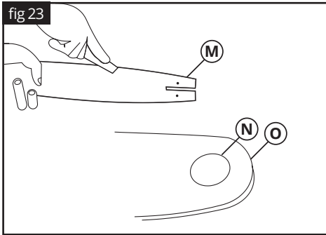
M. Oiling port / Οπή παροχής λαδιού N. Grease port / Είσοδος λίπανσης O. Sprocket / Οδοντωτός μηχανισμός
